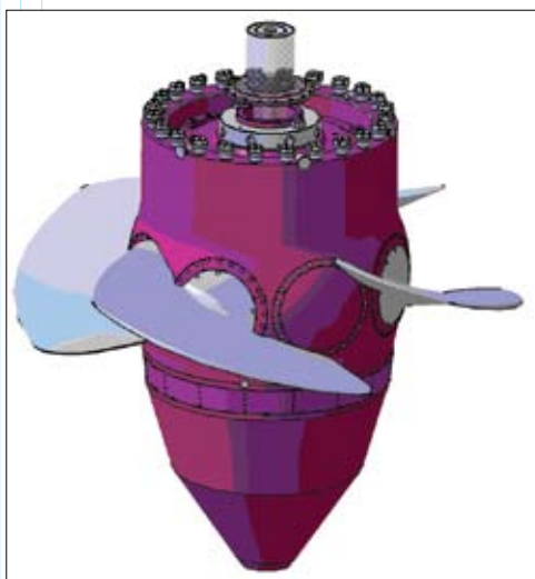
Рабочее колесо поворотной-лопастной турбины
