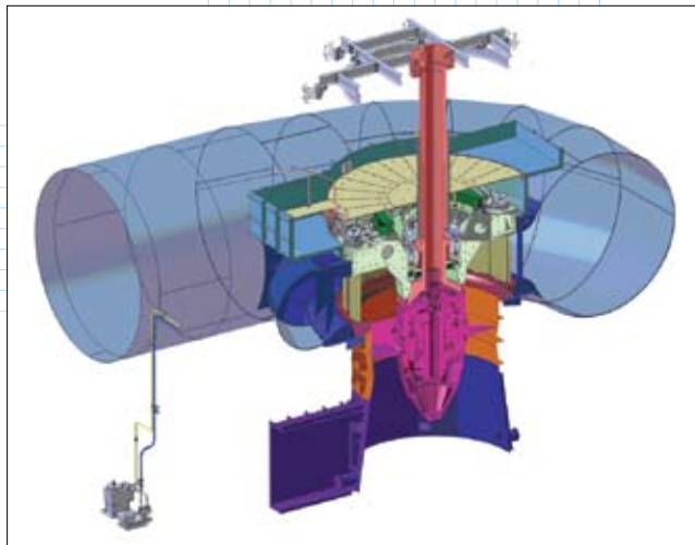
Сечение поворотной-лопастной турбины в сборе
