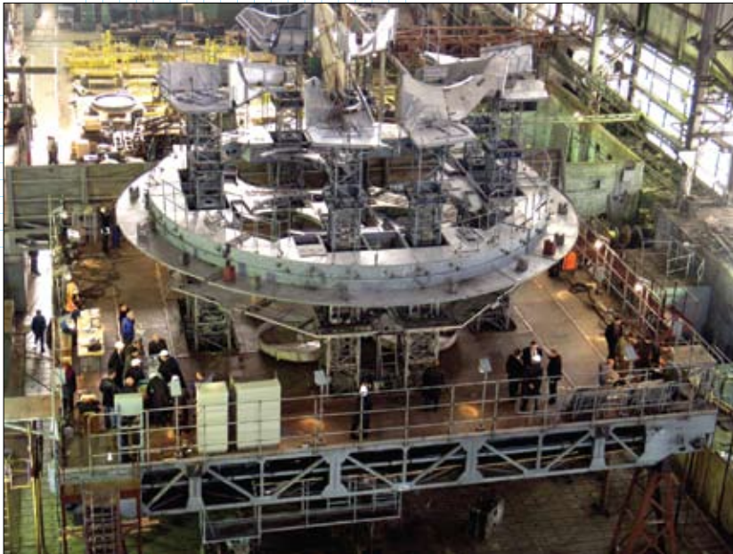
Кабина обслуживания для российско-французского космодрома Куру
